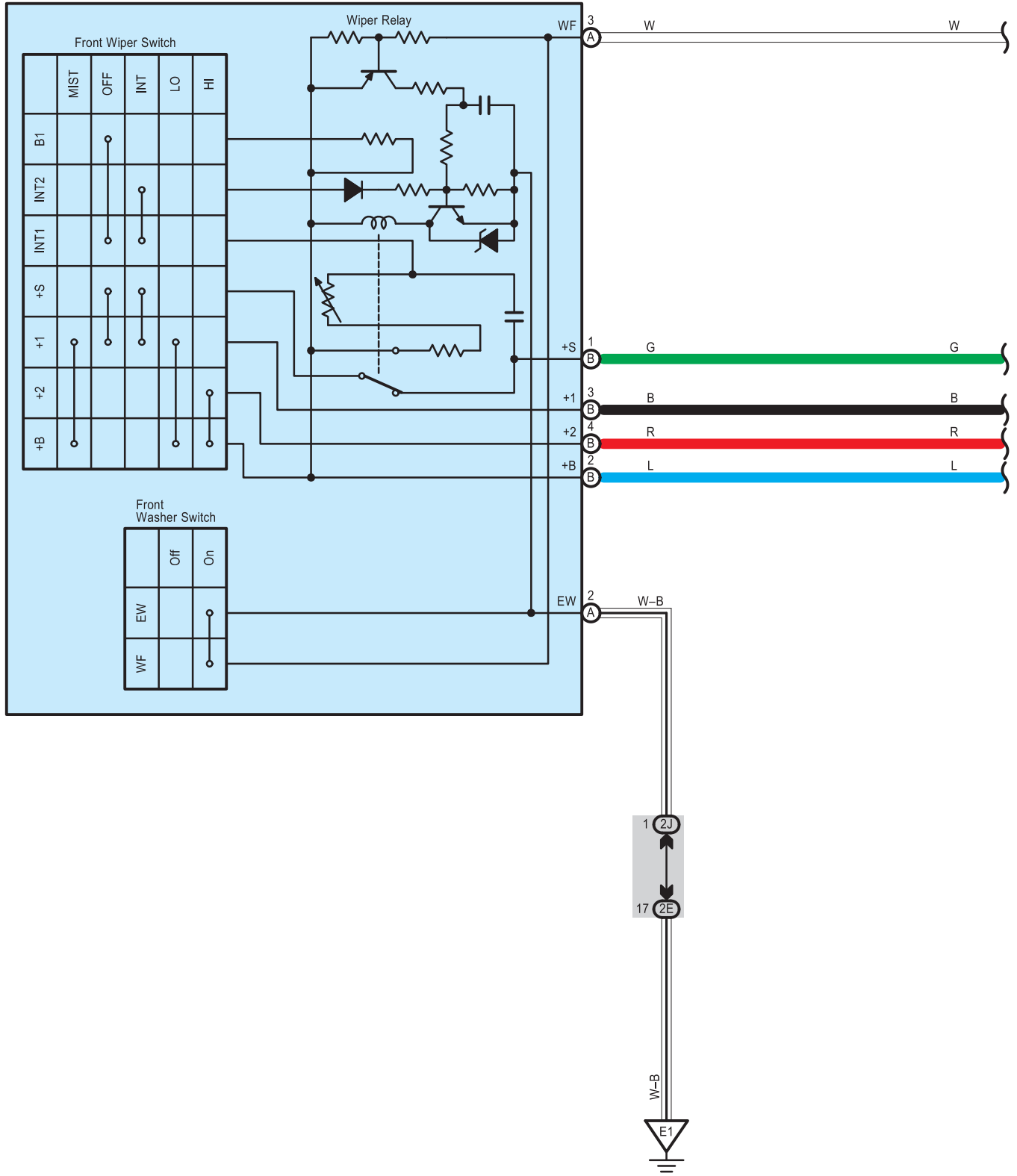
E9(A), E10(B) Windshield Wiper Switch Assembly
