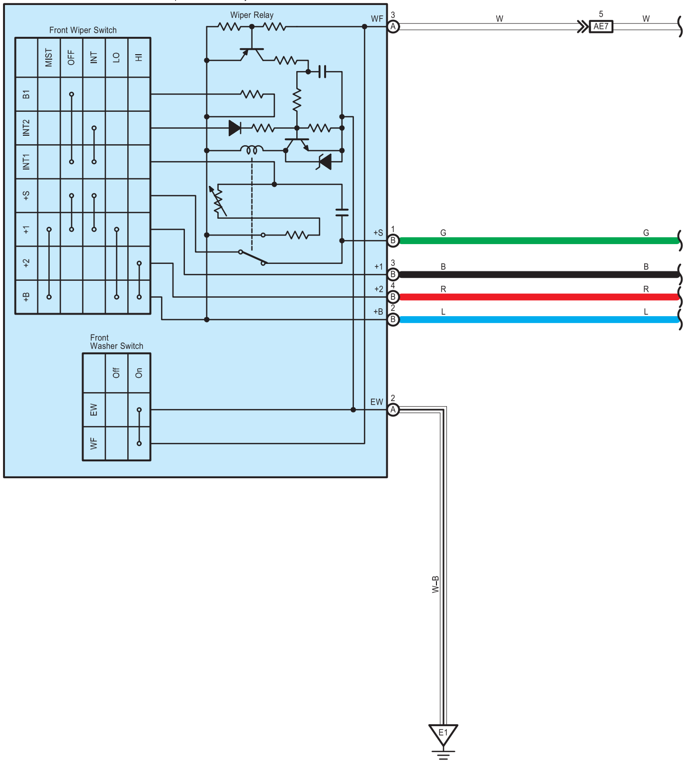
E9(A), E10(B) Windshield Wiper Switch Assembly
